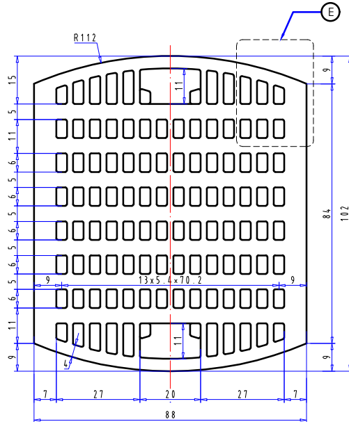
MẶT SAU ĐÌNH PHẦN QUANG
