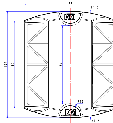
HÌNH CHIẾU ĐỨNG (KHÔNG DÁN PHẦN QUANG)
