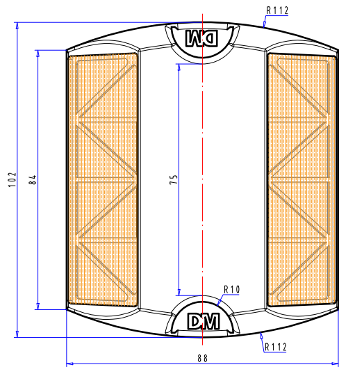
HÌNH CHIẾU ĐỨNG
