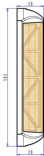
HÌNH CHIẾU CẠNH
