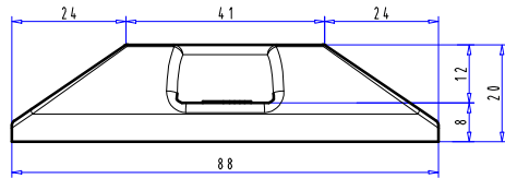
HÌNH CHIẾU BẰNG
