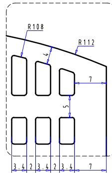
DETAIL E SC: 2:1
