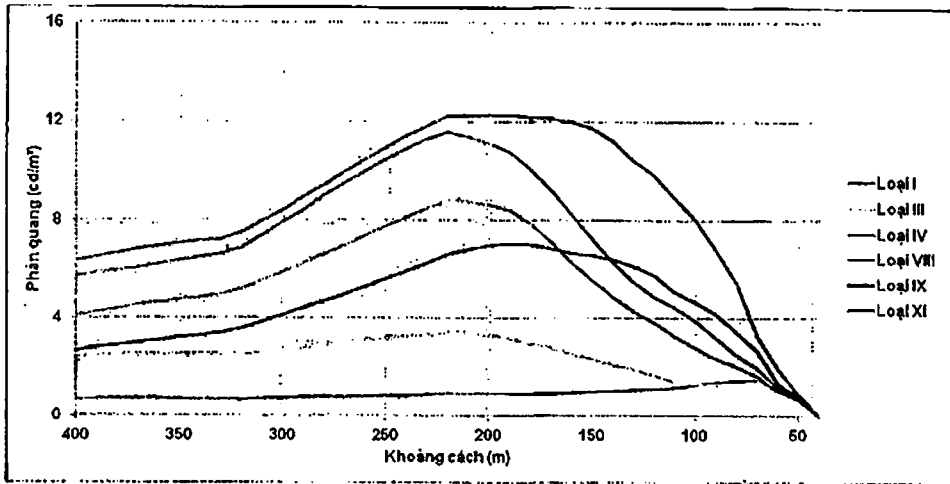
Hình E.6: Độ phân quang cầu biên báo đặt trên giá long môn đối với xe tải
